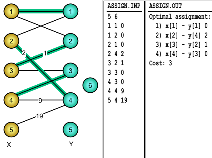
P_4_12_1.PAS * Thuật toán Hungari
